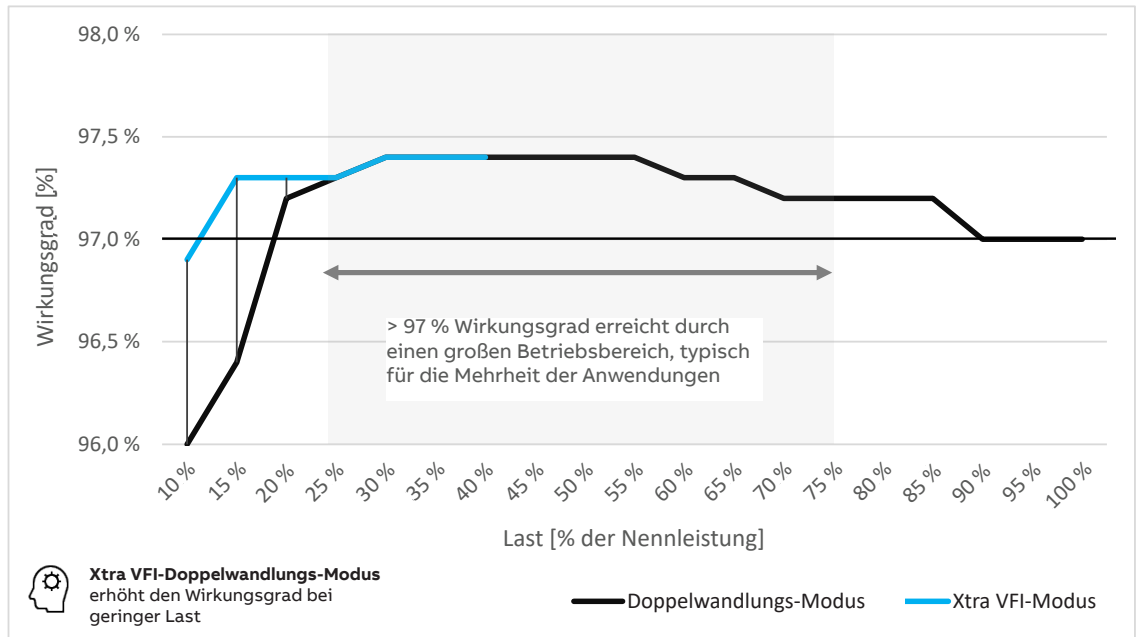
1.1-1: DPA 250 S4 Wirkungsdiagramm
